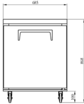
ELEVATION
